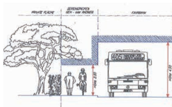
Freizuhaltenes Lichtraumprofil an öffentlichen Straßen, Wegen und Plätzen
